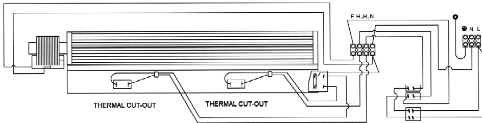
Fig 4 WIRING DIAGRAM - HE7420-31
